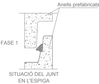
DETALL JUNT F-104
