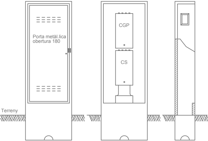
Soport prefabricat per C.G.P, 2 sortides i caixa seccionament (industrial)
