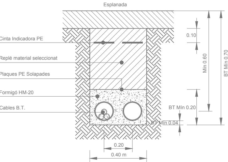
RASA TIPUS PER A ENTUBAR
