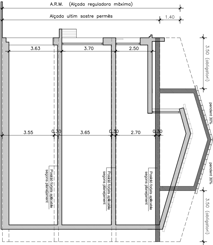
SECCIO
