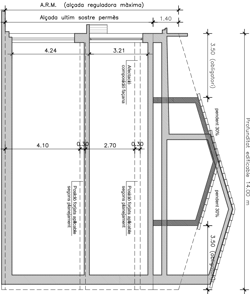
SECCIÓ ORIENTATIVA
