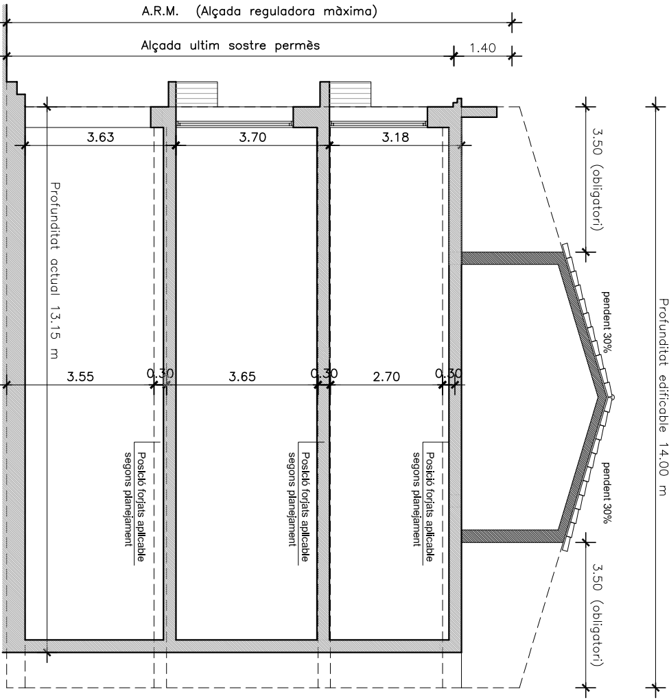
SECCIO
