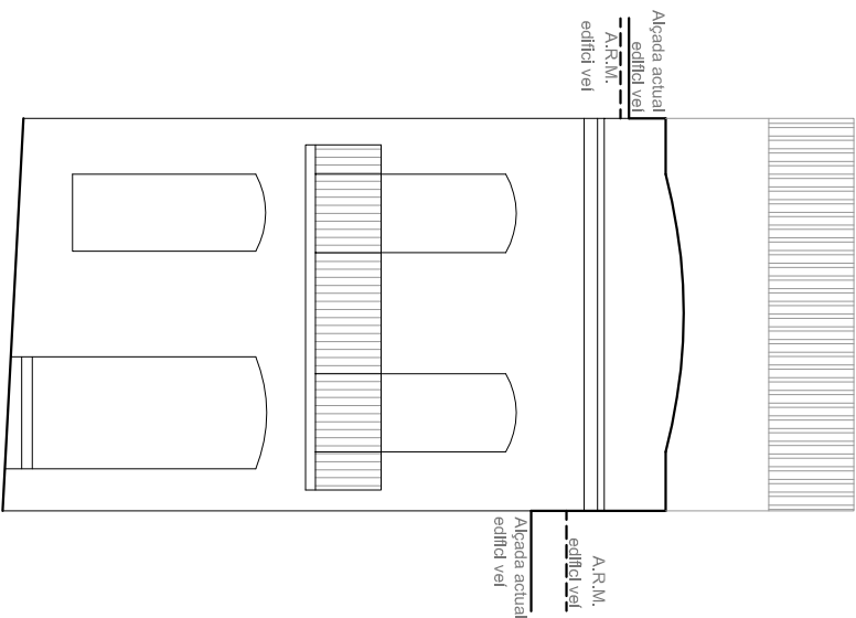
FAÇANA
