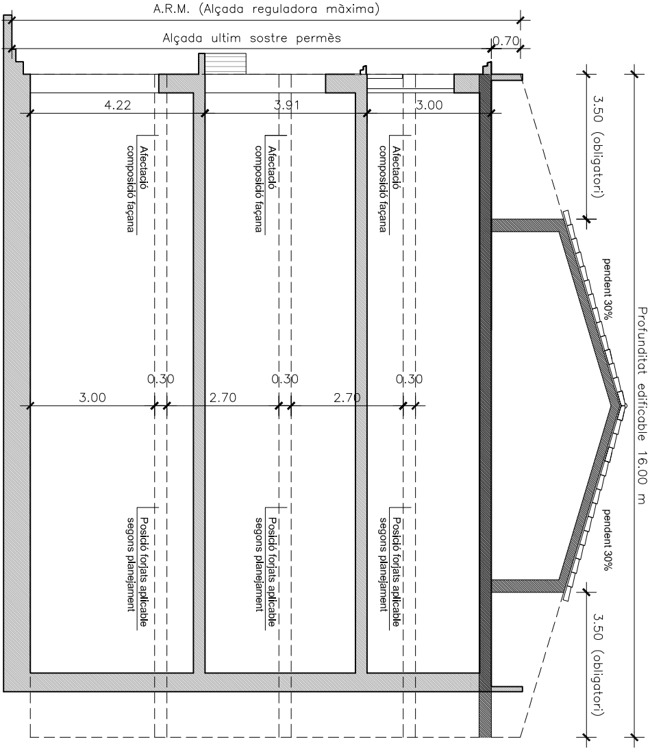
SECCIÓ ORIENTATIVA
