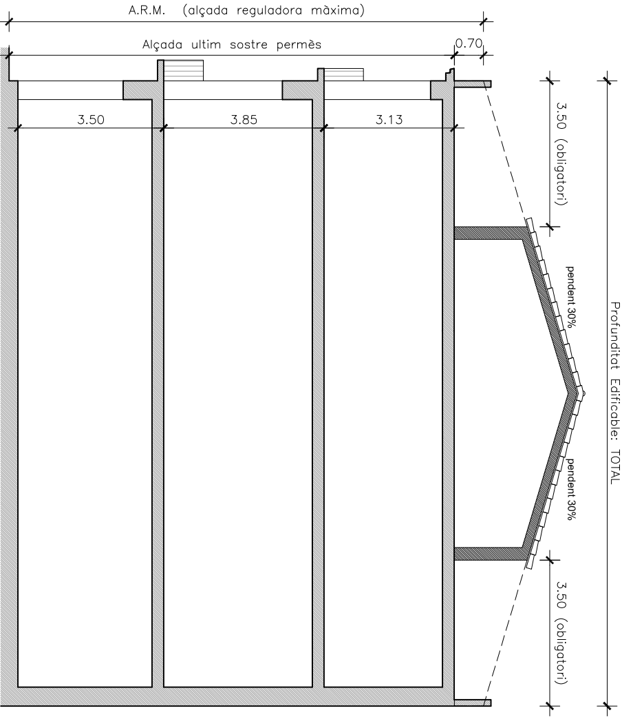
SECCIÓ ORIENTATIVA
