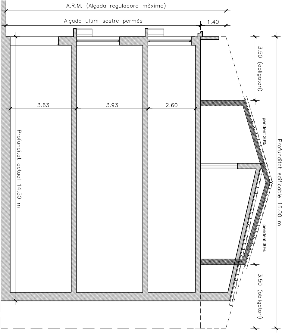
SECCIÓ
