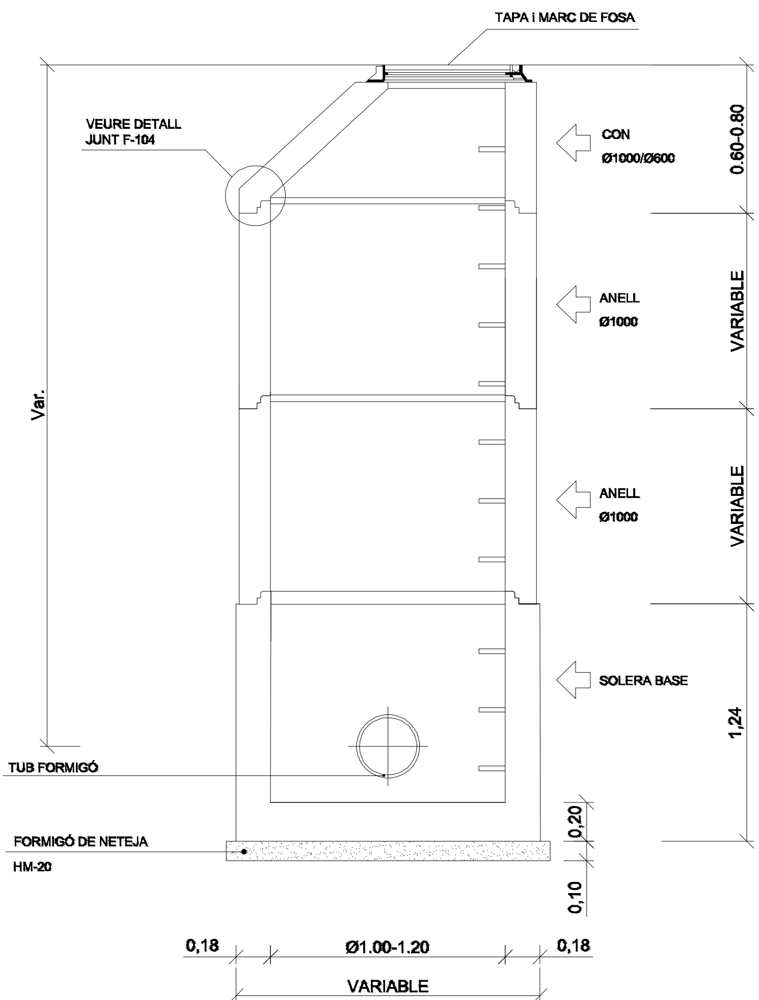
SECCIÓ A
