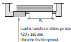
DETALLE PUERTA MARCO ANCHO
