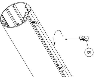
DETALL DE L'ENGANXAMENT DE LA XARXA
